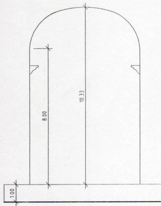
ALZADO ESCENARIO ESCALA= 1/100
